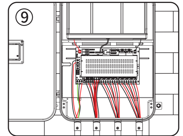
将电线或通信线从设备底部引入,并按接线图正确接线
