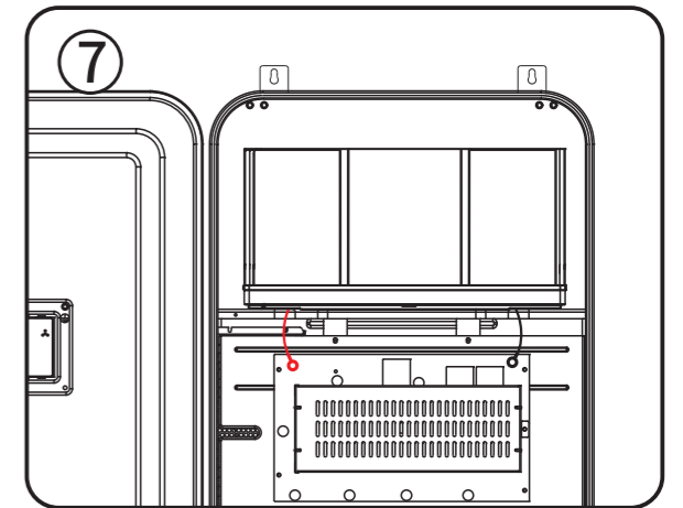
将备用电源装入箱内,注意备用电源需倒置安装,并且备用电源的正负极不得接反
