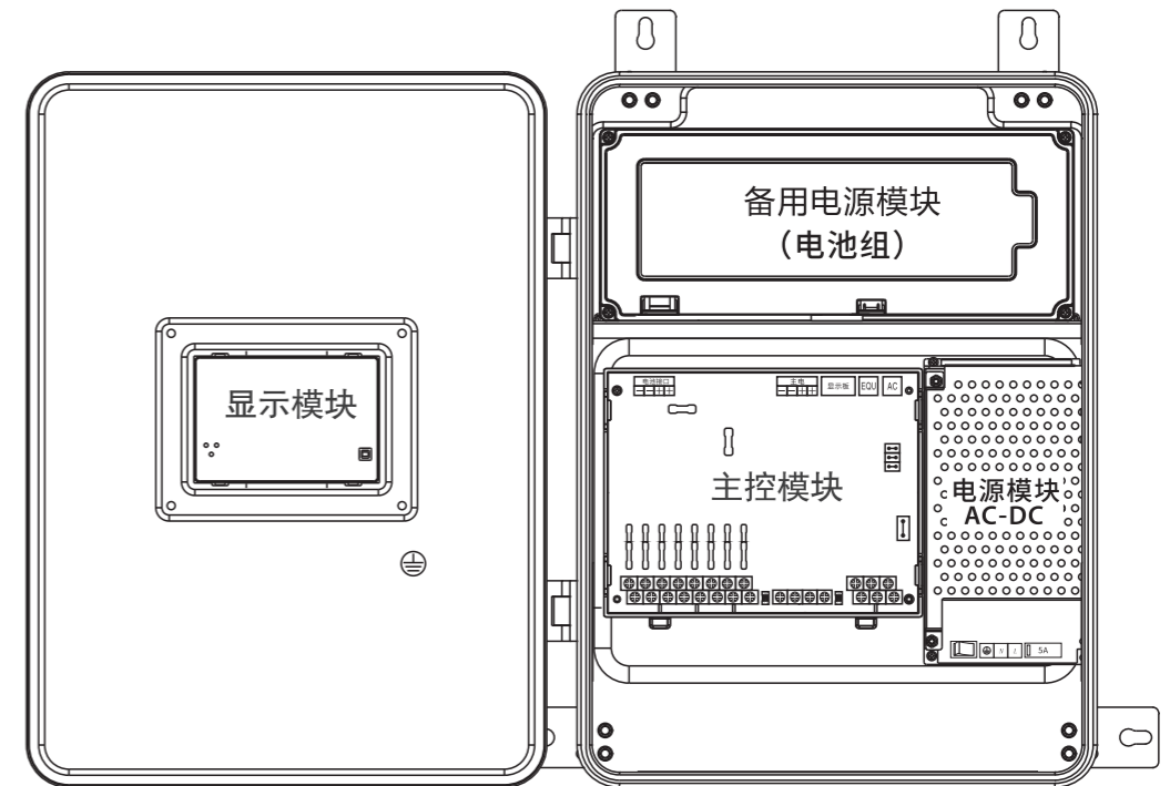
150W/200W 应急照明集中电源内部图
