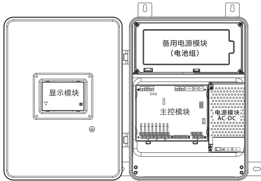
300W 应急照明集中电源内部图
