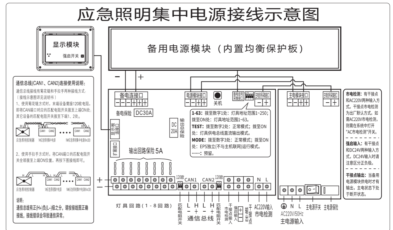
300W 应急照明集中电源接线示意图
