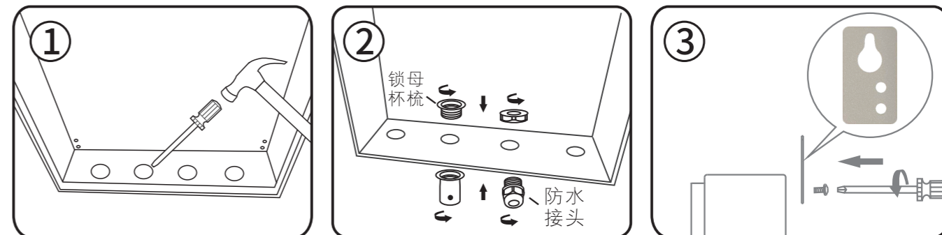
将箱体底部的预留孔撬出
