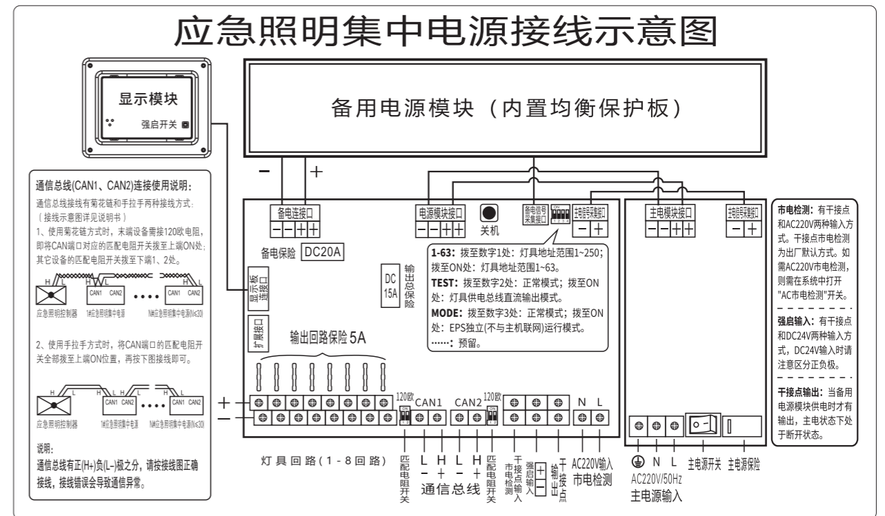
150/200W 应急照明集中电源接线示意图
