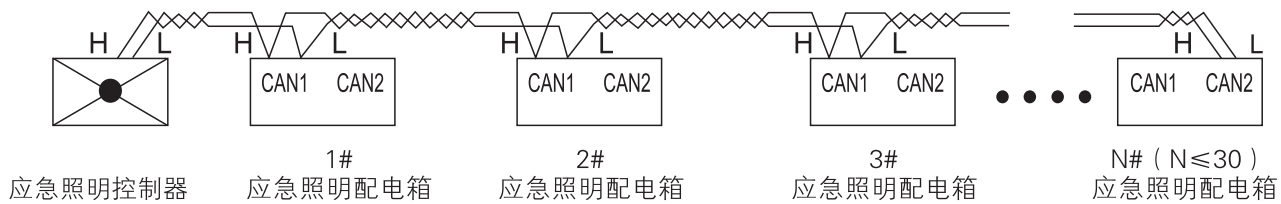
菊花链连接方式示意图（图2）
