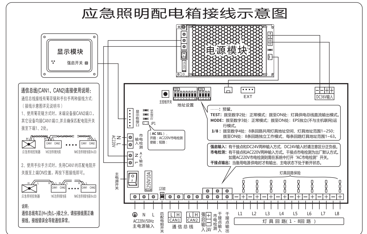
300W接线示意图 图4.3
