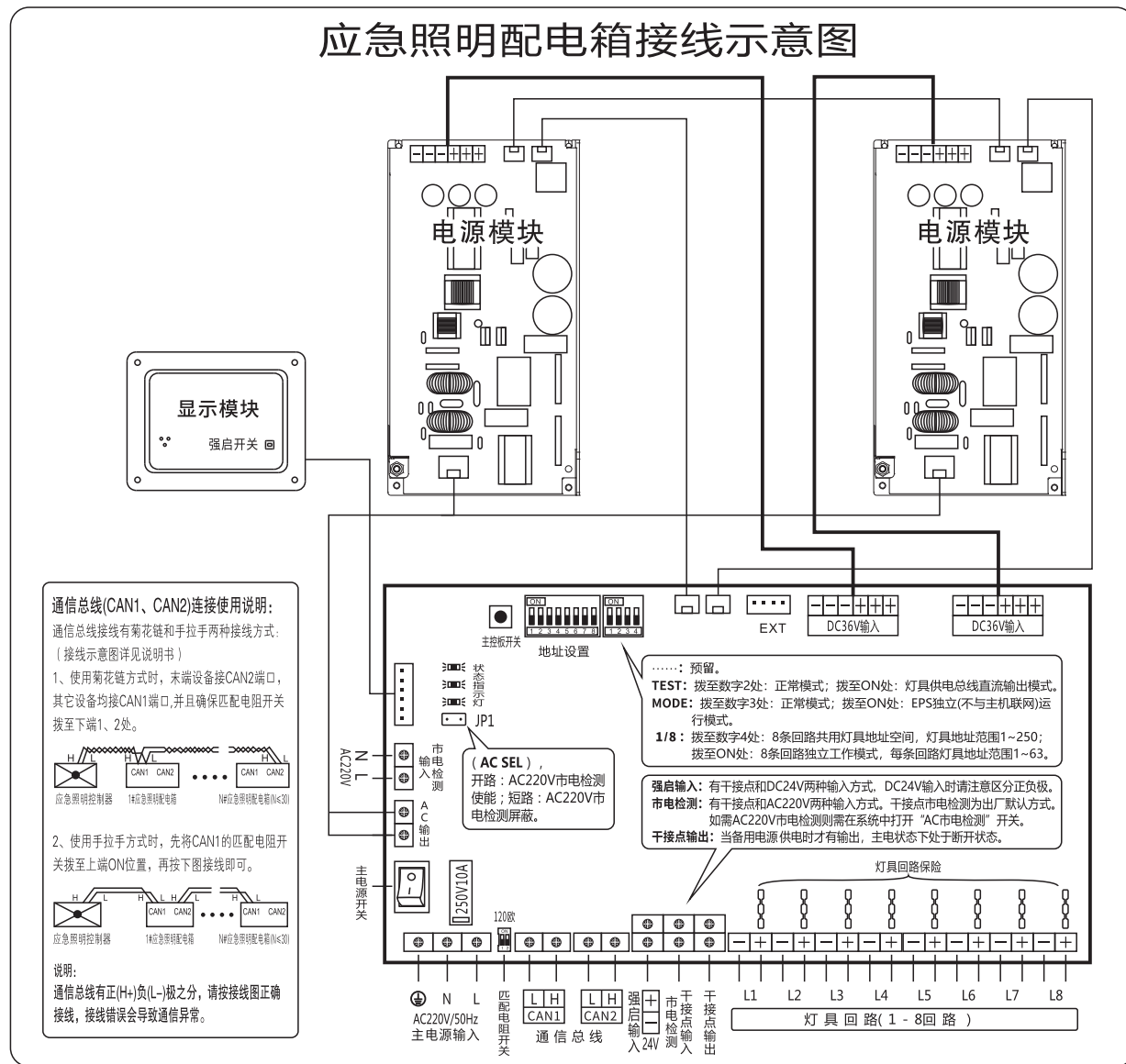
1000W接线示意图 图4.1
