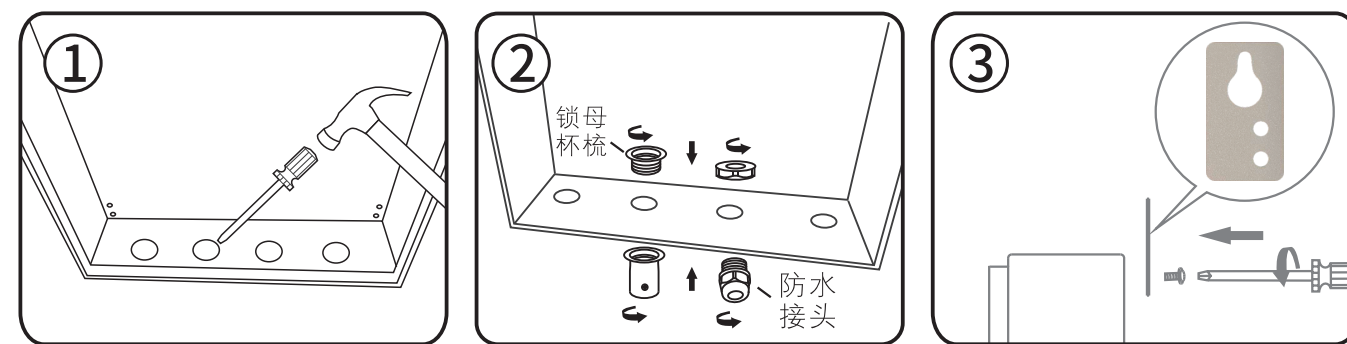
将箱体底部的预留孔撬出 将镀锌管锁母杯梳或防水接头 用螺丝刀将螺丝固定在机箱上装进开好的孔上
