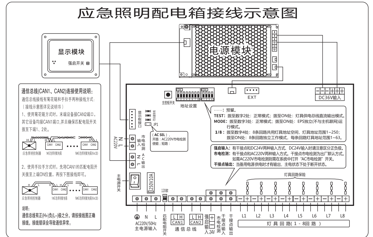
500W接线示意图 图4.2
